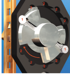
Pencere kolunu çevirirken yaylı emniyet pimleri [1] hassas bir klik sesiyle gövdedeki [2] özel aralıklara oturur.
