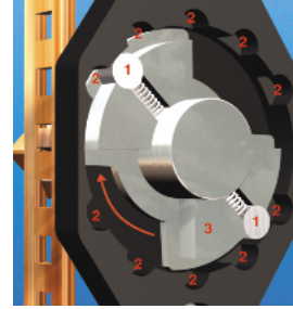
Dönüş hareketi sırasında emniyet pimleri [1] kavrama elemanından [3] diğer aralıklara [2] çekilir ve burada tekrar duyulur şekilde yerine oturur.
