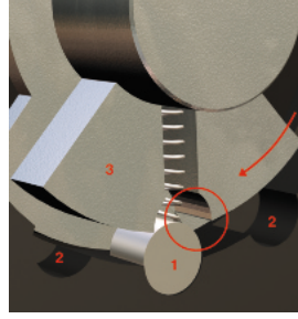
Hırsızlık girişimi sırasında emniyet pimleri [1] ikinci bir kavrama elemanı [3] tarafından gövdedeki [2] aralıklara bastırılır.
