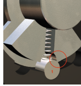
Bu konumda emniyet pimleri [1] pencere kolunun dıştan döndürülmesini etkili bir şekilde önler. Pencere kolu hırsızlık girişimini engeller ve önler.
